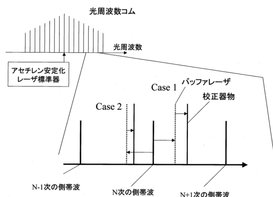
図4 式(1)に現れる周波数の値の関係を説明。
