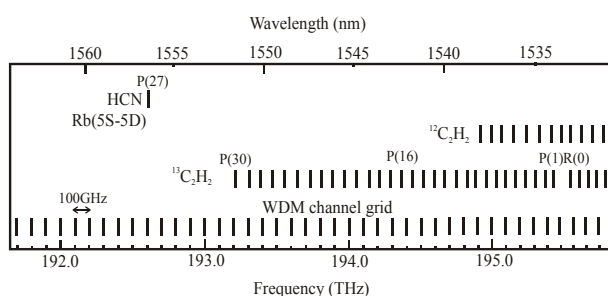
図1 ITU-Tの 100 GHz グリッド とアセチレンの吸収線
